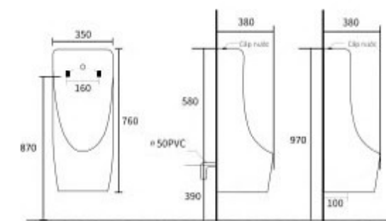
Thiết kế có thể xả ngang hoặc xả đáy linh hoạt
