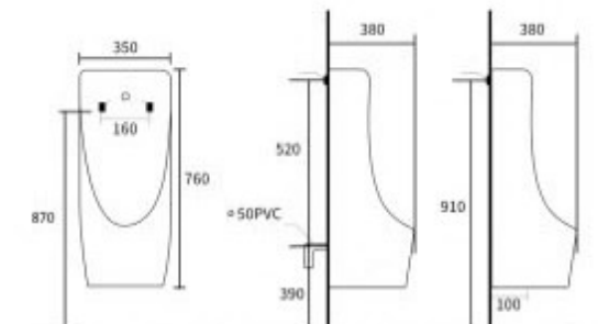
Thiết kế có thể xả ngang hoặc xả đáy linh hoạt
