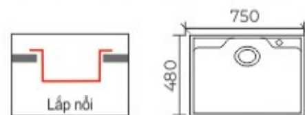
Bản vẽ, kích thước và cách lắp đặt
