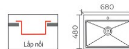
Bản vẽ, kích thước và cách lắp đặt
