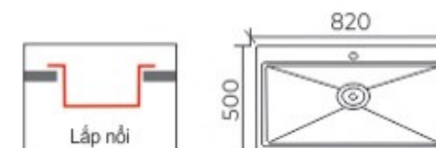
Bản vẽ, kích thước và cách lắp đặt
